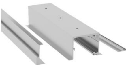
Conjunto perfil superior corredero FT . Montaje a falso techo. FT sliding top track set. False ceiling mounting. Set rail supérieur coulissant FT. Fixation à faux plafond.
